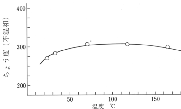
パイロノックユニバーサル2の温度-ちょう度関係
